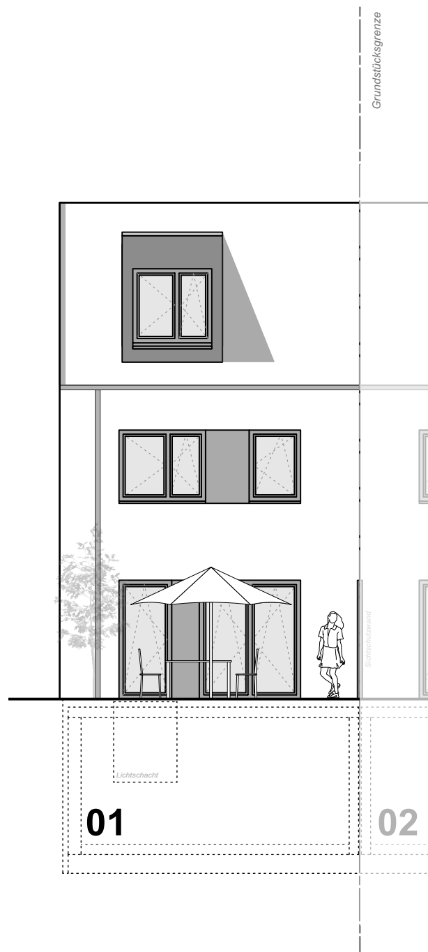
Ansicht Süd (Garten)
