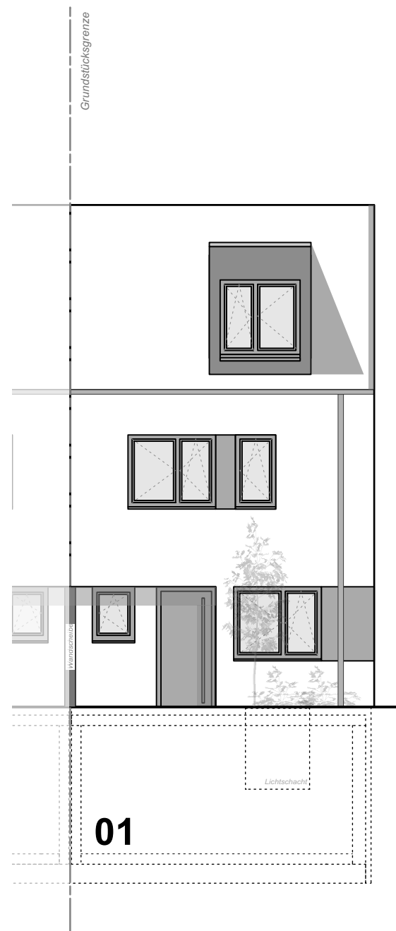
Ansicht Nord (Hauseingang)
